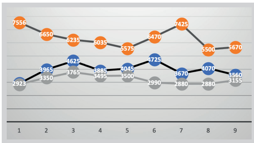
9. ábra. A Gongga-hegység gleccsereinek és régebbi végmorénáinak tengerszint feletti magassága (szerk. Mőga J.). Narancs görbe: a gleccserek felső határa (m); kék görbe: a gleccserek alsó határa (m); szürke görbe: a régebbi végmorénasáncok alsó határa (m). A gleccserek nevét a számozás alapján ld. a szövegben és az 1. táblázatban.
