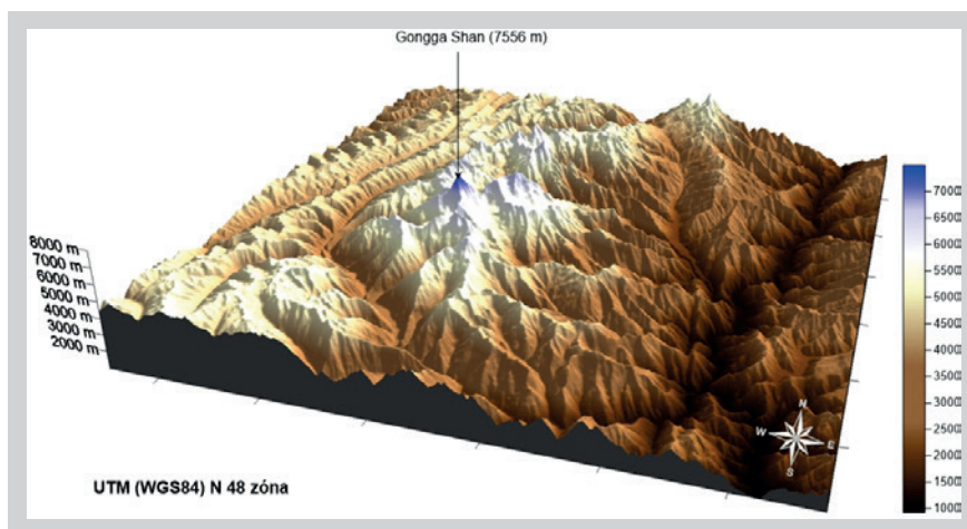
6. ábra. A Gongga-hegység tömbszelvénye (szerk. Cseri Z.). Jól látható a keleti és a nyugati oldal közötti aszimmetria.
