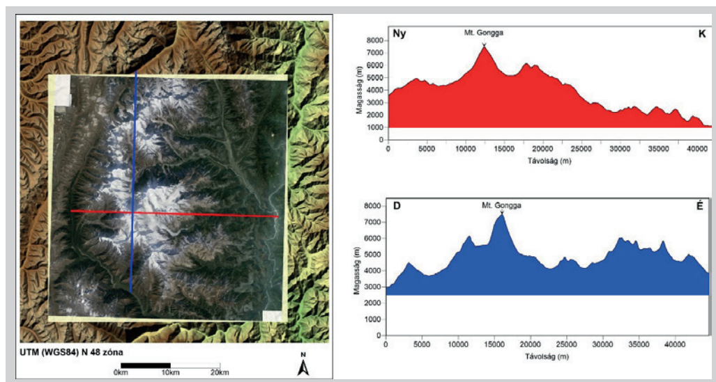
7. ábra. A Gongga-hegység területén készített nyugat-keleti irányú keresztmetszvény (szerk. Cseri Z.) jól érzékelteti a hegység aszimmetriáját. A keleti lejtőkön hosszú fehér völgyi gleccserek ereszkednek le, a nyugati oldalon morénával fedett sötétebb gleccserek figyelhetők meg.
